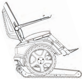
Raupenmodus
