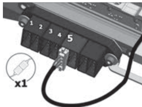
Abbildung 220. Die Verkabelung des Sitzneigemotors ist am Kontaktblock des Sitzrahmens angebracht.
