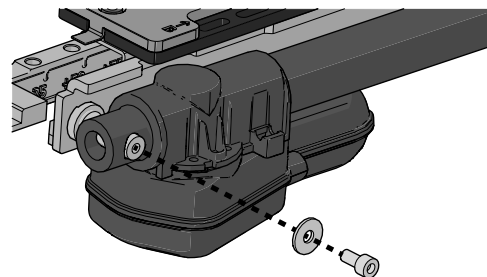
Abbildung 60. Vordere Befestigung der Stellvorrichtung.
