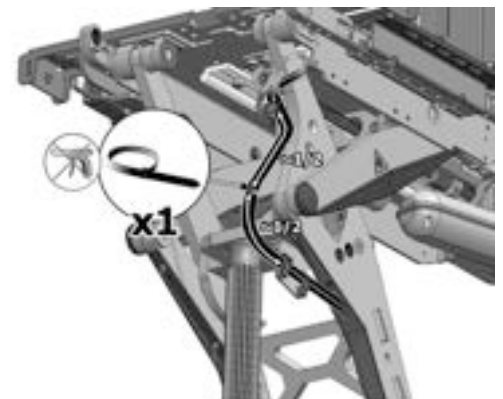
Abbildung 471. Die Buskabel R-net und ICS sind mit einem Kabelbinder in der Mitte der Kabelschleife miteinander verbunden.
