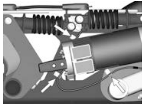
Abbildung 444. Das Kabel ist mit drei Kabelhalterungen auf der linken und rechten Seite des Fahrgestellkastens montiert.
