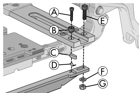
Abbildung 63. Die hintere Montage der Stellvorrichtungshalterung für die Rückenlehne.
