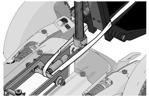
Abbildung 277. ... und die Achse an der unteren Rückseite der AP-Höhenverstellung an.
