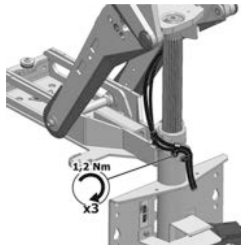
Abbildung 474. Das Kabel ist mit drei Kabelhalterungen an der Säule befestigt und jeweils mit einer Schraube montiert.
