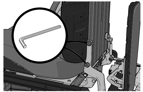
Abbildung 96. Das Profil der Rückenlehne ist mit zwei Schrauben links und rechts gesichert.
