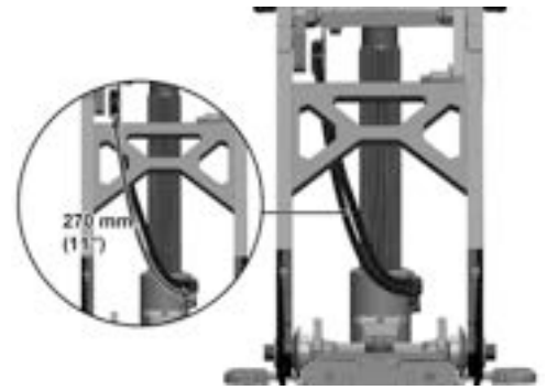
Abbildung 472. Die Länge der Kabelschleife zwischen den Kabelhalterungen am unteren Bereich der AP-Höhenverstellung und dem Pfosten muss 270 mm betragen.
