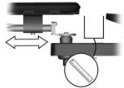
Abbildung 525. Einstellen der Position des Steuerpults auf den früheren Modellen des Parallelpulthalters.
