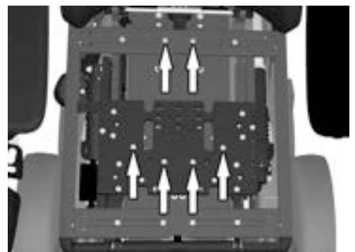
Abbildung 19. Der Sitz ist mit sechs Schrauben montiert.
