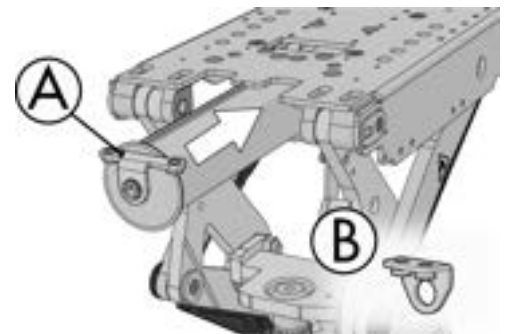
Abbildung 305. Drücken Sie das Kunststofflager auf die Spindel.
