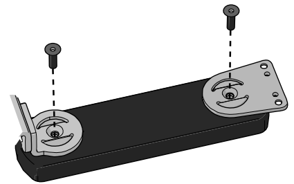
Abbildung 533. Die zwei Schrauben, mit denen die Platten gesichert werden.
