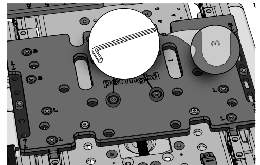
Abbildung 269. Position der zwei Bolzen.
