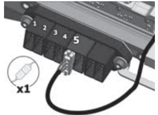
Abbildung 235. Die Verkabelung des Sitzneigungsmotors ist am Kontaktblock des Sitzrahmens angebracht.
