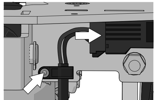
Abbildung 301. Schließen Sie das Kabel der Stellvorrichtung an.
