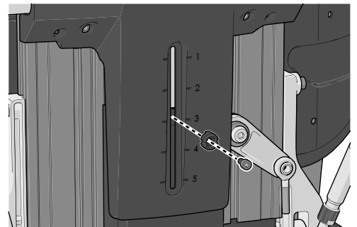
Abbildung 22. Der Kunststoffknopf ist mit einer Schraube befestigt.
