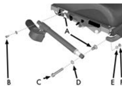
Abbildung 129. Die REAC-Stellvorrichtung für die Beinstütze wird von zwei Verschraubungen (B) und (C) gehalten.
