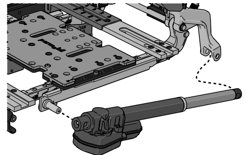
Abbildung 45. Die Stellvorrichtung muss herausgewinkelt werden.
