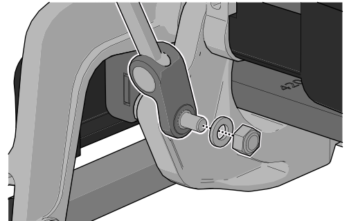
Abbildung 509. Halten Sie die Gelenkschraube fest, um die Mutter entfernen zu können.
