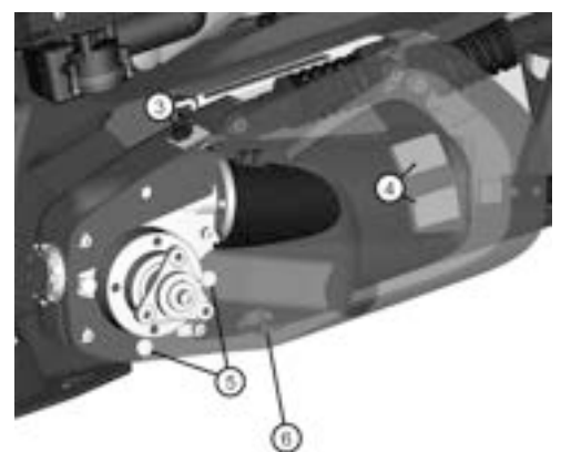
Abbildung 200. Die Antriebsmotor-Abdeckung ist mit Klettverschlüssen (3 - 4) und einem Befestigungspunkt (5) an der Unterseite angebracht.
