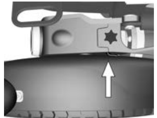
Abbildung 193. Ziehen Sie bei Rollstühlen mit Beleuchtung das Kabel aus dem Schlitz heraus, um Zugang zum Kabelstecker zu erhalten. Zerlegen Sie den Stecker, um die vordere Beleuchtung auszustecken.
