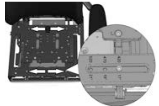
Abbildung 493. Die Sitzbreite ist mit vier Schrauben fixiert.
