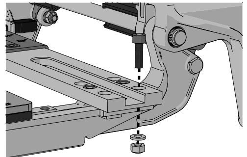
Abbildung 67. Die M6x20 Schraubenposition.
