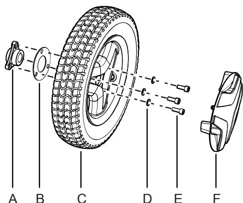
Abbildung 380. Montieren des Antriebsrads.
