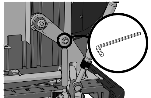
Abbildung 87. Das Gelenk für die Schiebefunktion der Rückenlehne ist mit einer Schraube befestigt.
