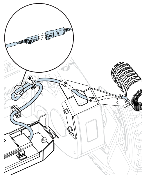
Abbildung 451. Ziehen Sie das Kabel aus den Schlitzen heraus und befestigen Sie es mit einem Kabelbinder, positionieren Sie dann das Ende des Beleuchtungskabels nach oben über die Bohrung durch den Kotflügel.
