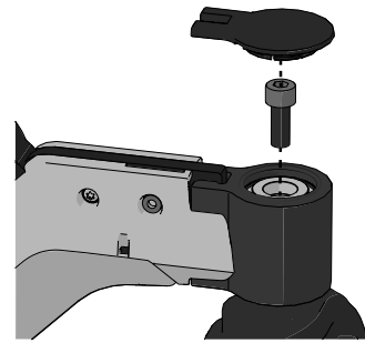
Abbildung 411. Entfernen Sie die Abdeckung und lösen Sie die Schraube.
