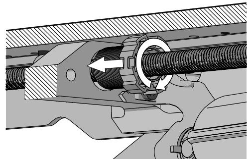
Abbildung 286. Schrauben Sie die Polymermutter in den Schlitten.
