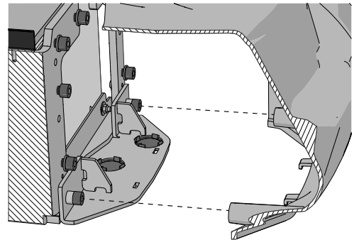
Abbildung 185. Die unteren Schrauben des Fahrgestellkastens müssen mit den Öffnungen an den Formstücken übereinstimmen.
