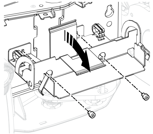
Abbildung 243. Halterung des ICS-Mastermoduls.
