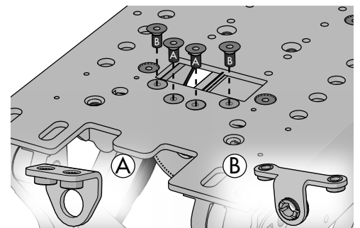
Abbildung 306. Es gibt verschiedene Bohrungen für die Schrauben, die je nach Halterungsversion variieren.
