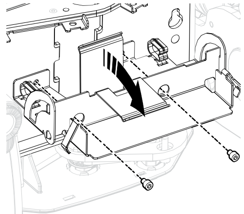
Abbildung 247. Halterung des ICS-Mastermoduls.
