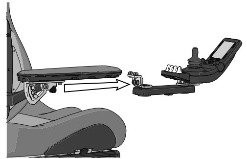
Abbildung 107. Der neue Parallelpulthalter ist mit zwei Muttern in der UniTrack angebracht.
