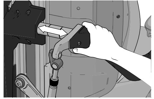
Abbildung 507. Es sind Markierungen auf der Achse vorhanden, um Sie bei der Ausrichtung zu unterstützen.
