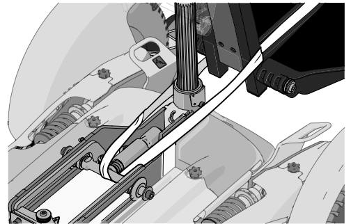
Abbildung 289. Lösen Sie die Achse an der unteren Rückseite der AP-Höhenverstellung.
