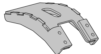
Abbildung 316. Rollhalterung.
