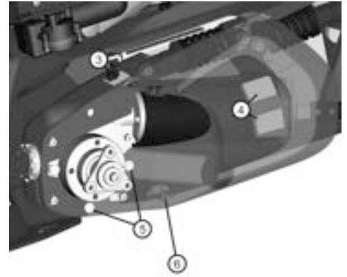
Abbildung 195. Die Antriebsmotor-Abdeckung ist mit einem Knauf (3) auf der Oberseite und einer doppelten Verriegelung (4) auf der Seite und einem Befestigungspunkt (5) an der Unterseite angebracht.
