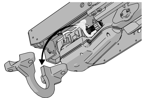
Abbildung 267. Entfernen Sie die Halterung.
