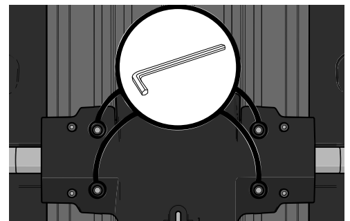
Abbildung 503. Einstellung der Armlehnenhöhe.
