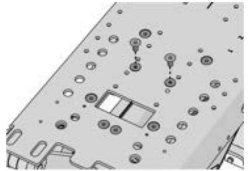
Abbildung 313. Position der zwei Bolzen.
