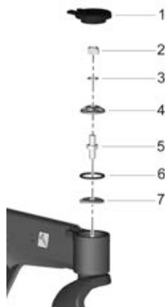
Abbildung 545. Reibungsbremse.
