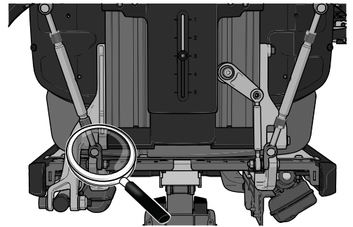
Abbildung 508. Der Anbringungsort der linken Einstellstange.
