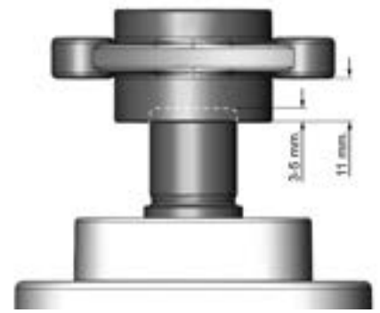
Abbildung 404. Sie müssen die Nabe mit der längeren Zwischenhülse (11 mm) des Getriebegehäuses passt.
