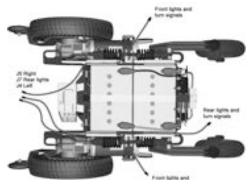
Abbildung 445. Beleuchtungsverkabelung.
