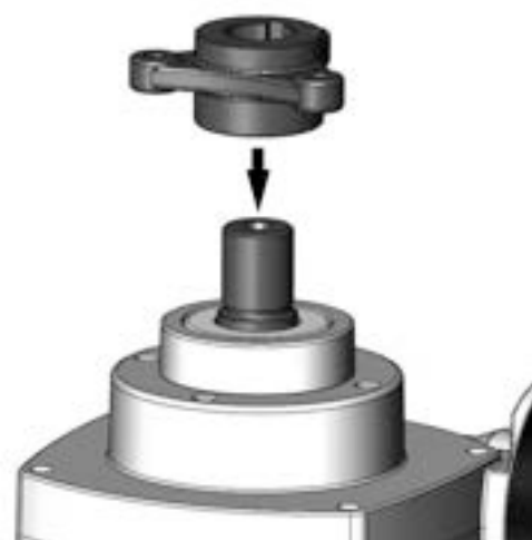
Abbildung 403. Positionieren Sie die Nabe auf der Achse.
