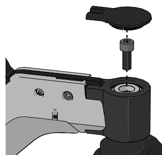
Abbildung 436. Schieben Sie die Abdeckung in ihre Position.
