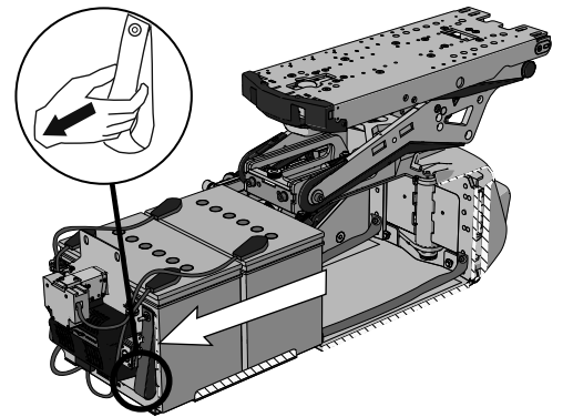
Abbildung 359. Bänder zum Herausziehen des Batteriekastens.
