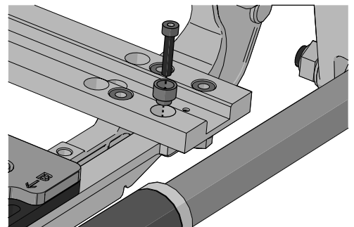
Abbildung 75. Die M4x20 Schraube durch die Buchse befestigen.
