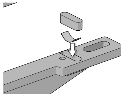
Abbildung 64. Blattfeder und Taste.
