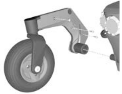
Abbildung 192. Die Gelenkarmabdeckungen sind mit drei Schrauben angebracht.
