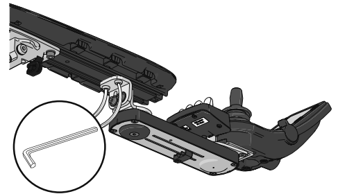
Abbildung 105. Die Position der Schrauben auf dem neuen Modell des Parallelpulthalters.
