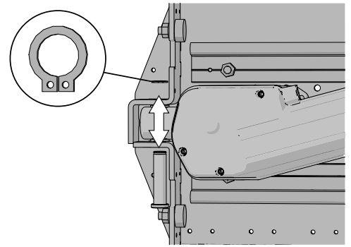
Abbildung 288. Bringen Sie den Sicherungsring und die Achse wieder an.
