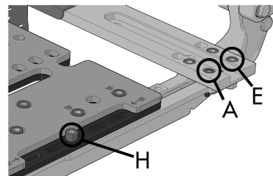
Abbildung 76. Die vordere Befestigung (H), M4x20-Schraube (A) mit der Buchse und M6x20 (E) mit der Unterlegscheibe und Sicherungsmutter an der hinteren Befestigung.
