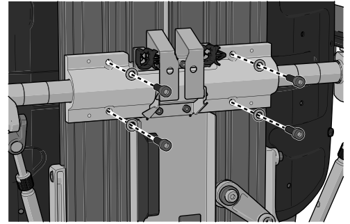
Abbildung 86. Die Armlehnen sind mit vier Schrauben befestigt.
