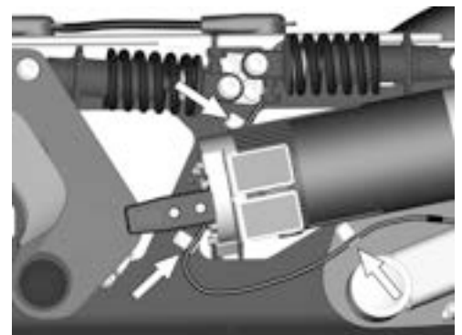
Abbildung 448. Das Kabel ist mit drei Kabelhalterungen auf der linken und rechten Seite des Fahrgestellkastens montiert.
