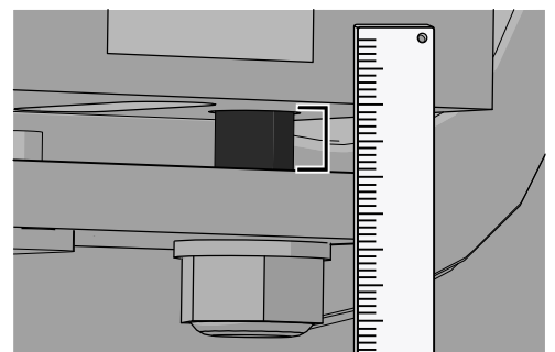
Abbildung 68. Die 1 mm Lücke zwischen der Stellvorrichtungshalterung und der hinteren Sitzstange.
