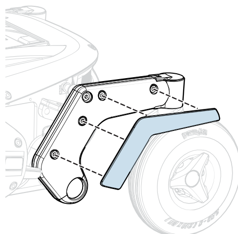
Abbildung 189. Gelenkarmabdeckung in Akzentfarbe.
