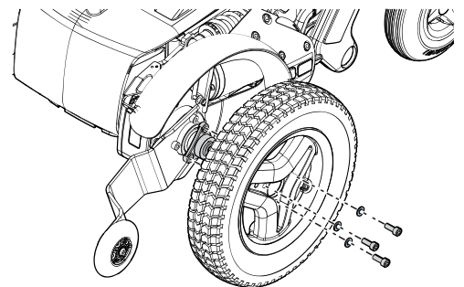
Abbildung 386. Ziehen Sie das Rad gerade heraus, nachdem Sie die drei Schrauben entfernt haben.
