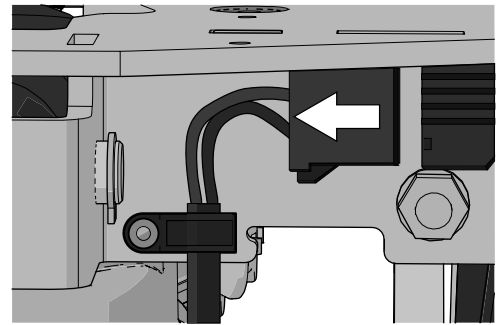
Abbildung 300. Trennen Sie das Kabel der Stellvorrichtung.
