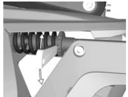
Abbildung 547. Verwenden Sie das Gerät, um die Federkraft anzupassen.
