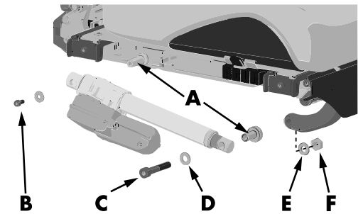
Abbildung 126. Die LINAK LA28-Stellvorrichtung für die Beinstütze wird von zwei Verschraubungen (B) und (C) gehalten.
