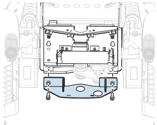
Abbildung 242. Entfernen Sie die Schutzplatte unter dem Motor.
