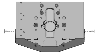
Abbildung 340. Die Kunststoffnieten befinden sich an den Seiten des Klemmschutzes.
