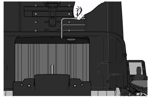
Abbildung 504. Der Schlüssel befindet sich in einer Vertiefung in der Rückenlehne.
