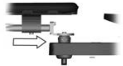
Abbildung 108. Das frühere Modell des Parallelpulthalters und der drehbare Pulthalter sind mit einer Klammer angebracht.
