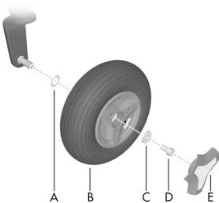
Abbildung 392. Zusammenbauen der Felge.
