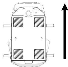
Abbildung 384. Position der Blöcke. Der Pfeil zeigt die Fahrtrichtung an.
