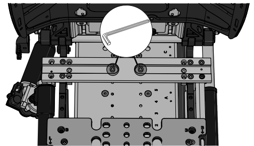
Abbildung 312. Position der zwei Bolzen.
