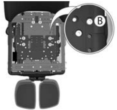
Abbildung 214. Die Position des hinteren Abschnitts des Sitzrahmens (Rückenlehnenposition) wird mit sieben Schrauben gehalten, die hier mit dem Buchstaben B markiert sind.
