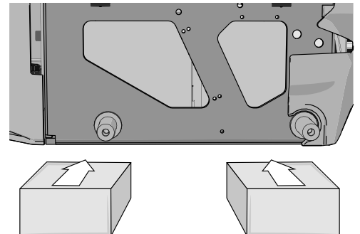
Abbildung 409. Verwenden Sie jeweils zwei Blöcke auf jeder Seite des Fahrgestellkastens. Zur besseren Darstellung wurden die Räder in dieser Abbildung entfernt.
