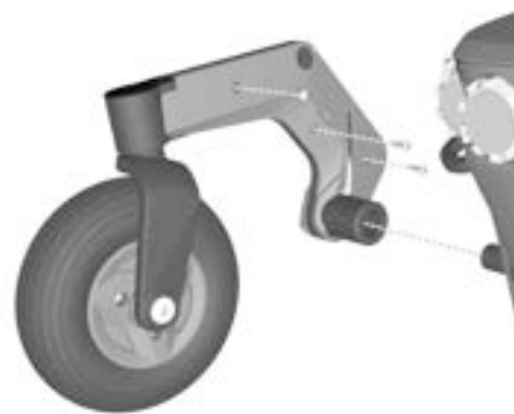
Abbildung 191. Die Gelenkarmabdeckungen sind mit drei Schrauben angebracht.
