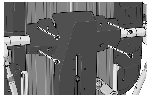
Abbildung 83. Die Anbringungsorte der vier Schrauben, die die Kunststoffabdeckung sichern.
