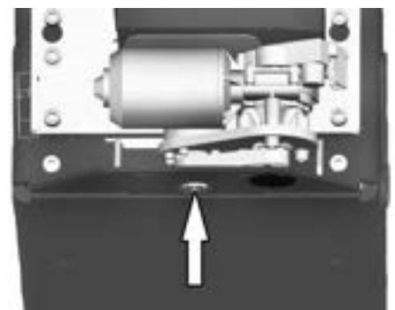
Abbildung 211. Entfernen Sie die Schutzabdeckung aus Gummi unter dem Fahrgestellkasten, um Zugang zur Achse der Sitzhöhenverstellung zu bekommen.
