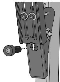
Abbildung 156. Verwenden Sie die M6x16-Schraube, um die Verriegelung zu sichern.
