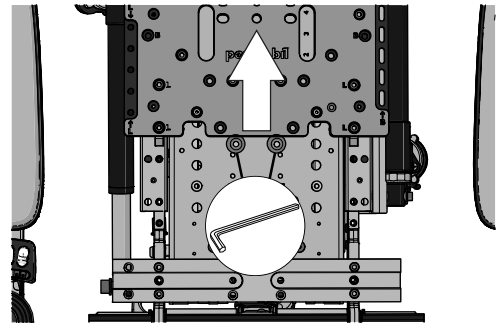
Abbildung 260. Je nach Sitztiefe muss möglicherweise ebenfalls die Rückenlehne bewegt werden.
