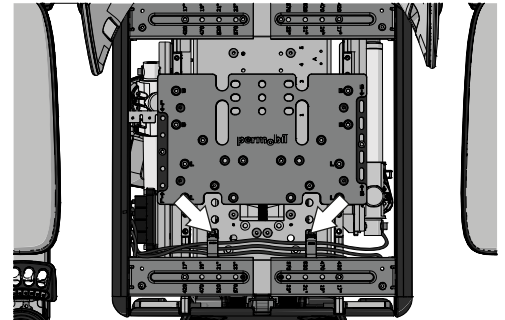
Abbildung 326. Die Position der Kabelclips.
