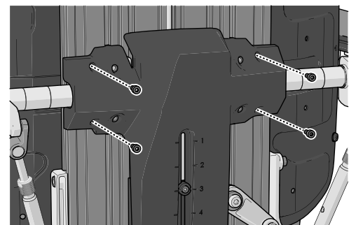
Abbildung 237. Die Anbringensorte der vier Schrauben, die die Kunststoffabdeckung sichern.
