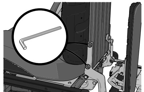
Abbildung 89. Das Profil der Rückenlehne ist mit zwei Schrauben links und rechts gesichert.
