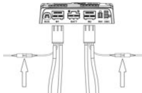
Abbildung 419. Verbinden der magnetischen Radsicherungen.
