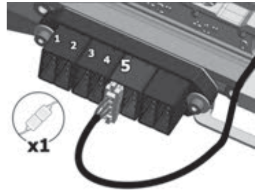
Abbildung 24. Das Motorkabel für die Sitzneigung befindet sich an der fünften Position des Verbinderblocks.
