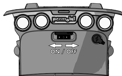
Abbildung 372. Hauptschalter unter dem Permobil-Logo auf der hinteren Abdeckung.
