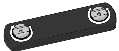
Abbildung 531. Die Verbindungsteile zur Einstellung weisen Zähne auf, die in ein entsprechendes Zahnpaar im Pulthalter eingreifen.
