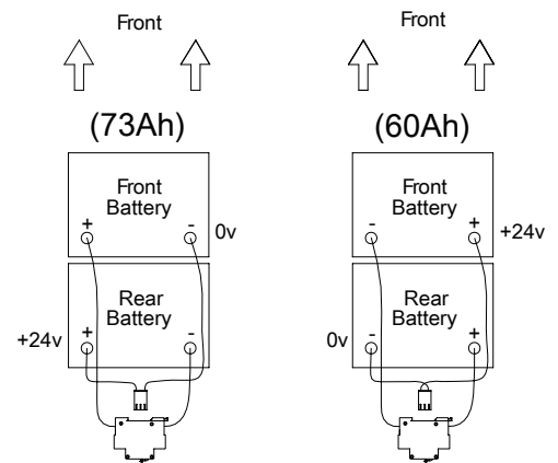
Abbildung 486. Batterieanschlüsse in Relation zur Batteriekapazität.
