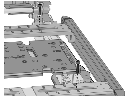
Abbildung 38. Die beiden Sitzplattenhalterungen sind mit zwei Schrauben befestigt.
