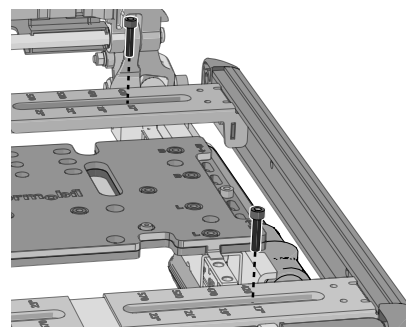
Abbildung 56. Die beiden Sitzplattenhalterungen sind mit zwei Schrauben befestigt.
