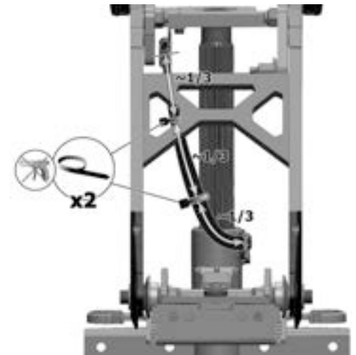
Abbildung 475. Die Buskabel sind in regelmäßigen Abständen per Kabelbinder an der Kabelschleife miteinander verbunden.
