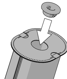
Abbildung 290. Setzen Sie das neue Kunststofflager in den Textilüberzug ein.
