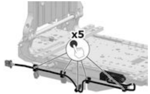
Abbildung 331. Das Kabel des Sitzneigungsmotors ist mit fünf Kabelhalterungen montiert (Sitztiefe 370 – 520 mm).
