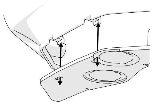
Abbildung 184. Schnapphaken und deren Befestigungspunkt im unteren Bereich des Fahrgestellkastens.
