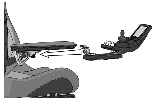
Abbildung 109. Der neue Parallelpulthalter ist mit zwei Muttern in der UniTrack angebracht.
