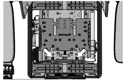
Abbildung 253. Die Position der Kabelclips wird mit den weißen Pfeilen markiert.
