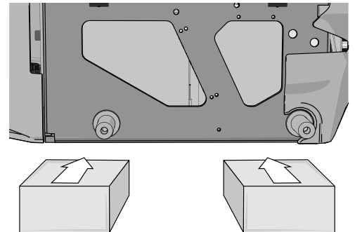
Abbildung 383. Verwenden Sie jeweils zwei Blöcke auf jeder Seite des Fahrgestellkastens. Zur besseren Darstellung wurden die Räder in dieser Abbildung entfernt.
