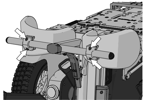
Abbildung 170. Auf jeder Halterung sind zwei Schrauben.
