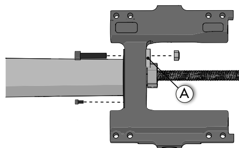
Abbildung 280. Schlitten A mit M6-Schraube und Mutter.
