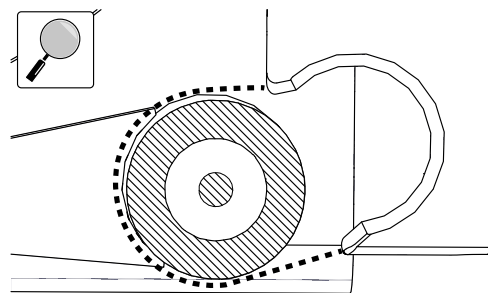
Abbildung 356. Über die Hinterachse hinausreichende Verlängerung der hinteren Abdeckung.
