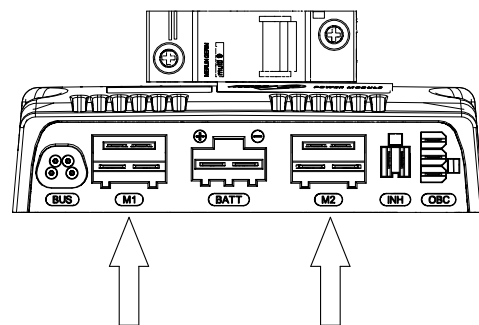
Abbildung 379. Verbinden Sie die Verkabelung von Magnetbremse und Antriebsmotor mit dem Leistungsmodul.
