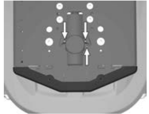
Abbildung 213. Der Elektromotor für den Sitzneigungsmechanismus wird mit drei Schrauben montiert.
