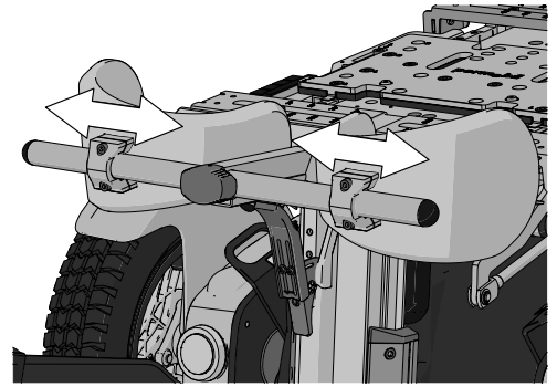
Abbildung 169. Es sollte problemlos möglich sein, die Halterungen zu verschieben, lösen Sie anderenfalls die Schrauben noch mehr.
