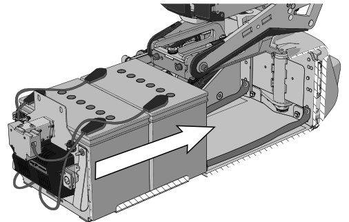
Abbildung 365. Schieben Sie den Batteriekasten hinein.
