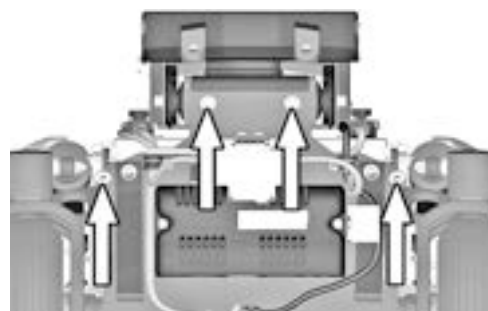
Abbildung 357. Der Batteriekasten ist mit vier Schrauben befestigt.
