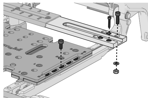
Abbildung 62. Entfernen Sie die drei Schrauben.
