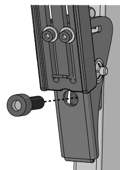
Abbildung 151. Die Verriegelung ist mit einer Schraube angebracht.
