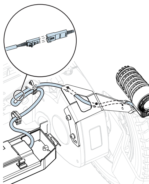
Abbildung 202. Bei Rollstühlen mit Beleuchtung müssen Sie sicherstellen, dass das Ende des Beleuchtungskabels nach oben über die Bohrung durch den Kotflügel verläuft.
