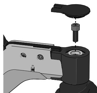
Abbildung 416. Schieben Sie die Abdeckung in ihre Position.
