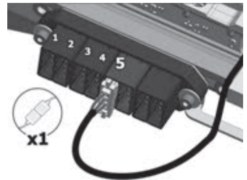
Abbildung 11. Das Kabel für den Sitzneigungsmotor befindet sich an der fünften Position des Verbinderblocks.
