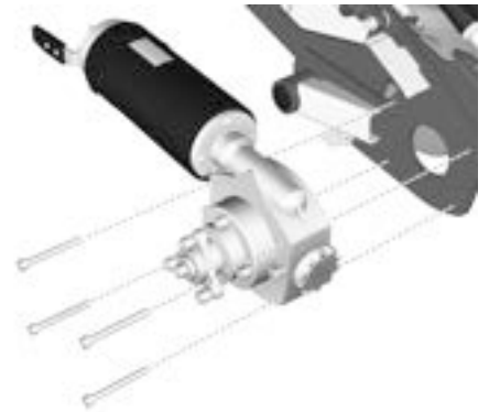
Abbildung 375. Anbringen oder Ausbauen des Antriebsmotors.
