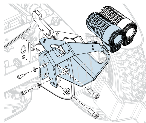
Abbildung 452. Die vordere Beleuchtung Sie ist mit zwei Schrauben von der Unterseite aus angebracht.
