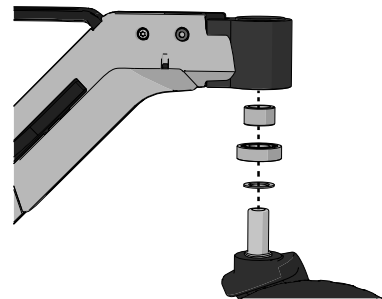
Abbildung 412. Abstandsstück, Lager, Unterlegscheibe und Radgabel.
