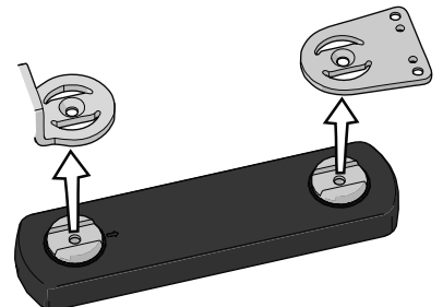
Abbildung 530. Die zwei Platten.
