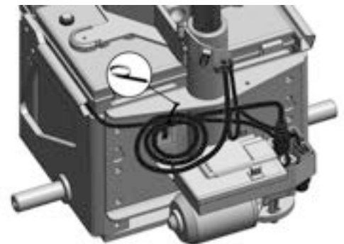
Abbildung 477. Der Rest der Kabel ist mit einem Kabelbinder zusammengebunden.
