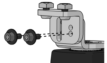
Abbildung 534. Die zwei Schrauben mit Unterlegscheiben auf dem neuen Parallelpulthaler.
