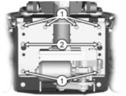
Abbildung 231. Die AP-Höhenverstellung ist vorn mit acht Schrauben befestigt.
