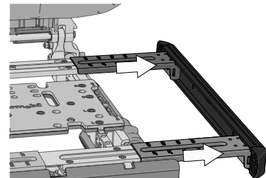
Abbildung 39. Die Halterungen können sich verkeilen, wenn Sie nicht beide gleichzeitig herausziehen.
