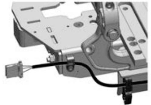
Abbildung 330. Die Position der beiden Kabelhalterungen.
