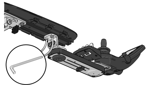
Abbildung 522. Die Position der Schrauben auf dem neuen Modell des Parallelpulthalters.
