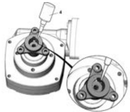
Abbildung 405. Tragen Sie eine dünne Schicht Loctite 638 um die Fasse der Achse auf.
