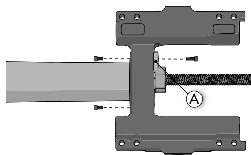
Abbildung 281. Schlitten B mit den M5-Schrauben.
