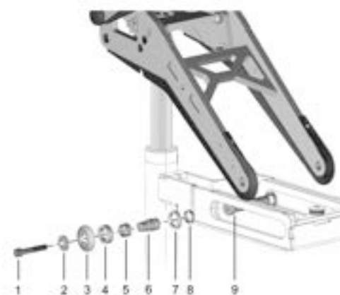
Abbildung 350. Laufradsatz.
