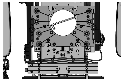
Abbildung 271. Position der zehn Bolzen.
