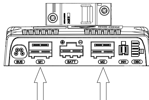
Abbildung 373. Trennen Sie die Magnetbremsen- und Antriebsmotor-Verkabelung vom Leistungsmodul.
