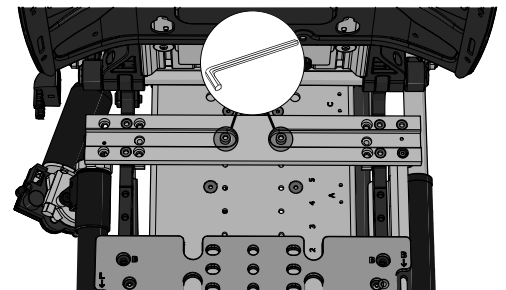
Abbildung 270. Position der zwei Bolzen.
