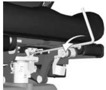
Abbildung 212. Verwenden Sie den Inbusschlüssel von der Rückenlehne aus, um manuell die Höhe der Sitzhöhenverstellung anzupassen. Der Sitz wird ohne die Beinstütze gezeigt, damit Sie eine bessere Sicht haben, die Beinstütze muss für diesen Vorgang nicht entfernt werden.
