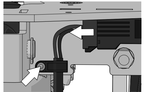
Abbildung 278. Rückansicht der oberen Platte der AP-Höhenverstellung.
