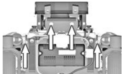
Abbildung 367. Der Batteriekasten ist mit vier Schrauben befestigt.
