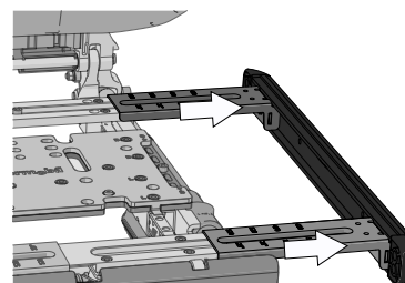
Abbildung 57. Die Halterungen können sich verkeilen, wenn Sie nicht beide gleichzeitig herausziehen.
