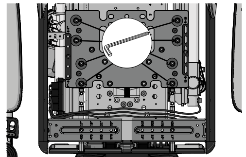
Abbildung 255. Position der acht Bolzen.
