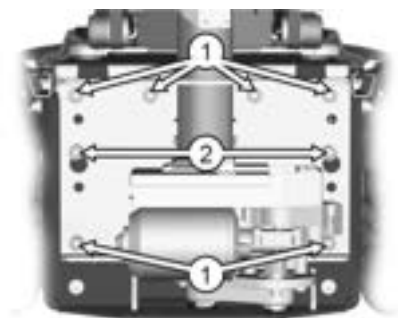
Abbildung 228. Die AP-Höhenverstellung ist vorn mit acht Schrauben befestigt.
