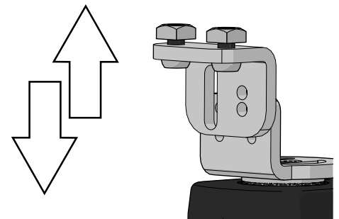
Abbildung 537. Höheneinstellung.
