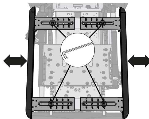
Abbildung 324. Position der vier Bolzen.
