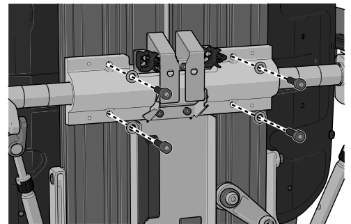
Abbildung 97. Die Armlehnen sind mit vier Schrauben befestigt.
