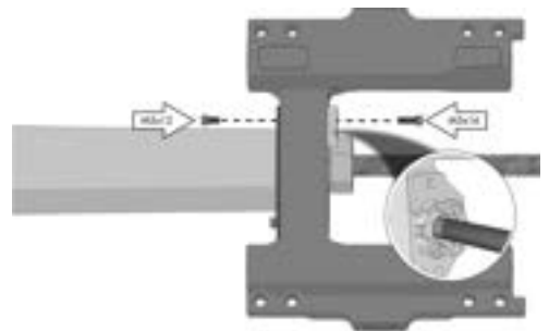
Abbildung 298. Schlitten B.
