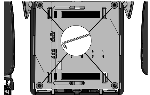
Abbildung 327. Die Position der vier Schrauben an der Sitzplatte.
