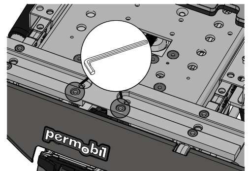
Abbildung 315. Position der zwei Bolzen.
