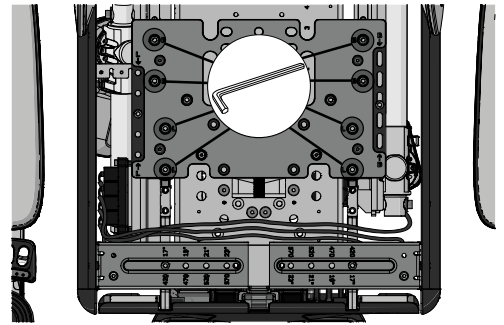
Abbildung 310. Position der acht Bolzen.
