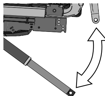
Abbildung 50. Bringen Sie die Stellvorrichtung in Position.
