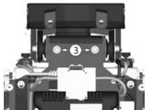
Abbildung 232. Die beiden Schrauben befestigen die AP-Höhenverstellung hinten.
