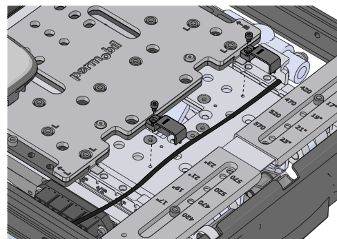
Abbildung 467. Das ICS-Buskabel wird über den Sitzrahmen verlegt und an den beiden Kabelhalterungen befestigt.
