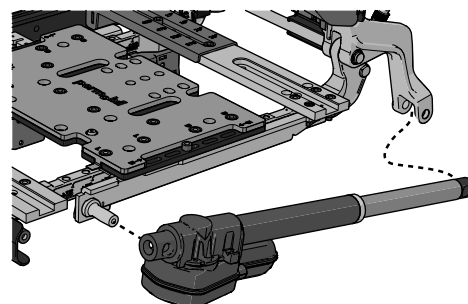
Abbildung 61. Die Stellvorrichtung muss herausgewinkelt werden.
