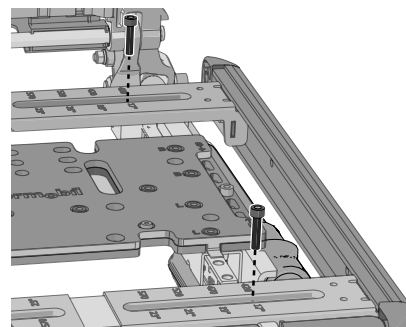
Abbildung 77. Die UniTrack-Schienenhalterungen werden mit zwei Schrauben befestigt.
