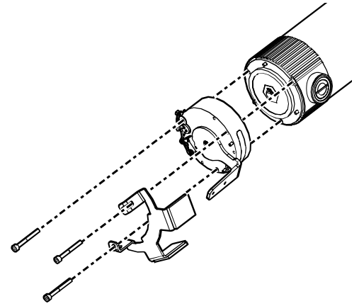
Abbildung 421. Die Magnetbremse ist mit drei Schrauben angebracht.
