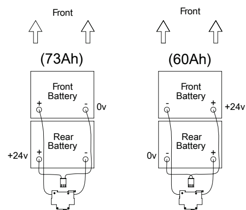
Abbildung 488. Batterieanschlüsse in Relation zur Batteriekapazität.
