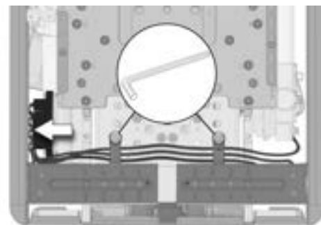
Abbildung 58. Stellvorrichtung Rückenlehne Verkabelung.
