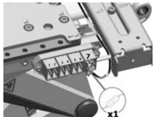
Abbildung 23. Das ICS-Buskabel befindet sich an der siebten Position des Verbinderblocks.
