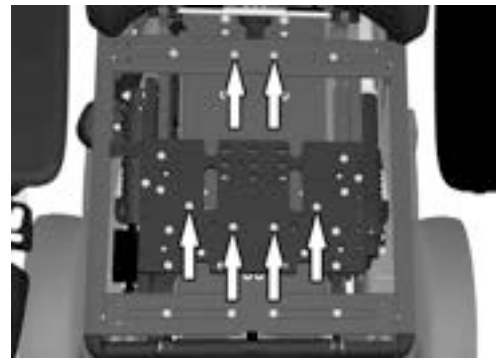
Abbildung 17. Der Sitz ist mit sechs Schrauben montiert.
