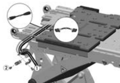
Abbildung 468. Der Abstand zwischen der ersten Kabelhalterung auf der AP-Höhenverstellung und dem Sitzrahmen muss 170 mm sein.
