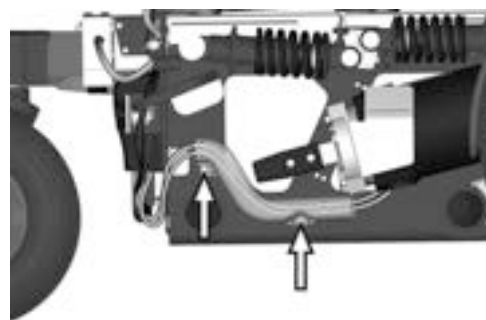
Abbildung 374. Die Kabel von Antriebsmotor und Magnetbremse werden mit einer Kabelabdeckung an ihrem Anbringungsort gehalten.
