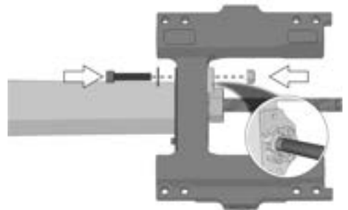
Abbildung 297. Schlitten A.
