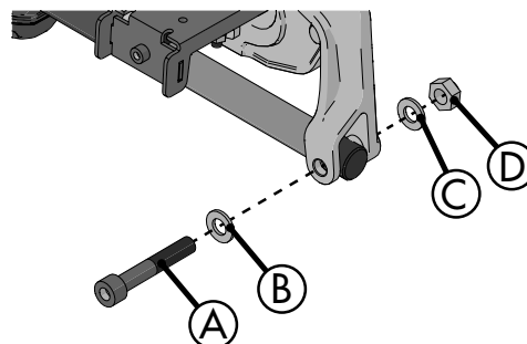
Abbildung 51. Hintere Befestigung der Stellvorrichtung.
