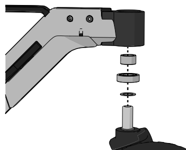
Abbildung 414. Abstandsstück, Lager, Unterlegscheibe und Radgabel.
