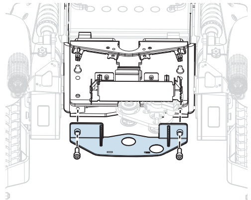
Abbildung 250. Befestigen Sie die Schutzplatte unter dem Motor.
