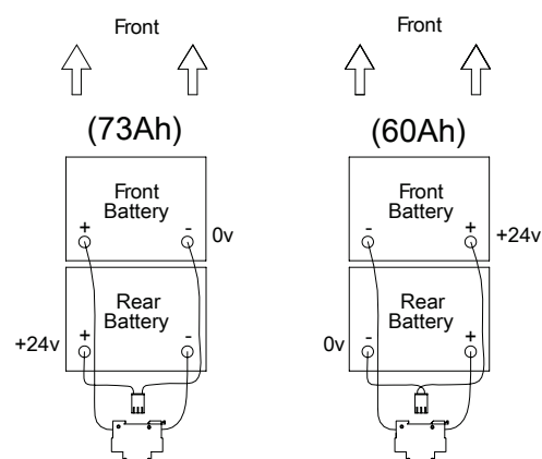
Abbildung 362. Schaltplan für den Batterieanschluss.
