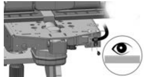
Abbildung 329. Die Kabelhalterung ist mit dem Kabelmantel montiert und steht ca. 5 mm vor.
