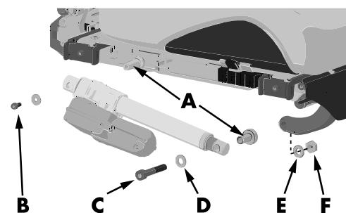
Abbildung 128. Die LINAK LA28-Stellvorrichtung für die Beinstütze wird von zwei Verschraubungen (B) und (C) gehalten.
