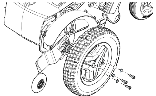
Abbildung 387. Bringen Sie das Rad auf der Radnabe an.
