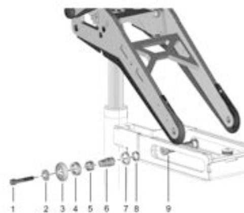
Abbildung 349. Laufradsatz.
