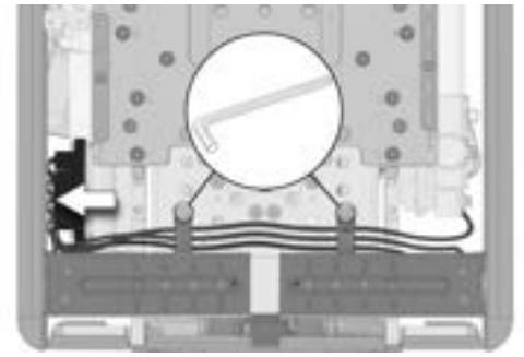
Abbildung 40. Stellvorrichtung Rückenlehne Verkabelung.
