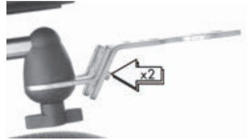
Abbildung 517. Die zwei Schrauben sichern den vorderen Teil des Pulthalters.
