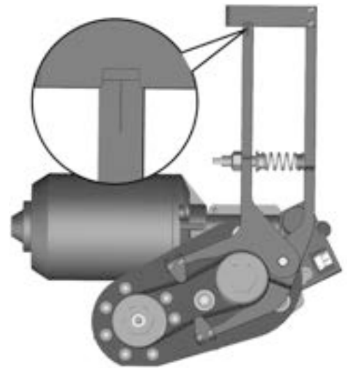
Abbildung 246. Die Zeigermarke befindet sich im erlaubten Bereich zwischen den Markierungen „links“ und „rechts“.
