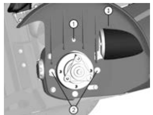
Abbildung 194. Der vordere Kotflügel ist mit einer Schraube (1) und zwei Befestigungspunkten (2) an der Unterseite angebracht. Der Rollstuhl wird ohne Antriebsrad gezeigt, damit Sie den vorderen Kotflügel besser sehen können. Das Antriebsrad muss für diesen Vorgang NICHT entfernt werden.
