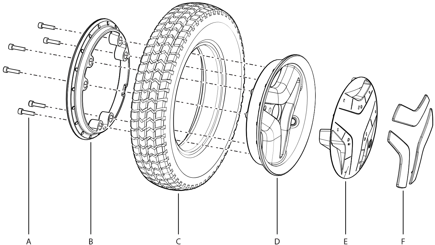
Abbildung 390. Anbringung oder Ausbau von Vollgummireifen oder Luftreifen.
