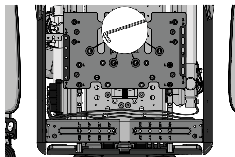
Abbildung 323. Position der vier Bolzen.
