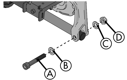
Abbildung 41. Hintere Befestigung der Stellvorrichtung.
