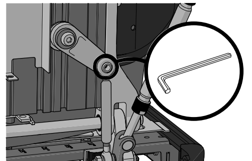
Abbildung 98. Das Gelenk für die Schiebefunktion der Rückenlehne ist mit einer Schraube befestigt.
