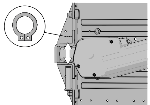
Abbildung 279. Entfernen Sie den Sicherungsring von der Achse.
