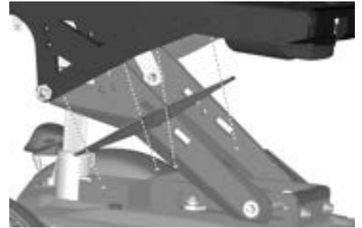
Abbildung 335. Der Klemmschutz ist mit vier Schrauben montiert.
