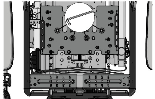
Abbildung 311. Position der vier Bolzen.
