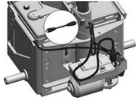
Abbildung 476. Die Buskabel sind mit dem ICS-Mastermodul verbunden.
