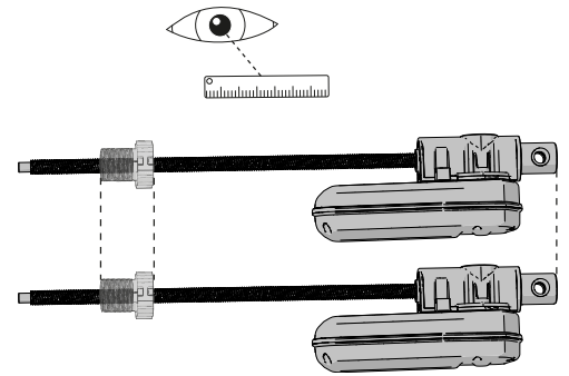
Abbildung 284. Positionieren Sie die neue Stellvorrichtung neben der alten.
