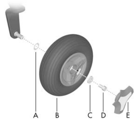
Abbildung 398. Zusammenbauen der Felge.
