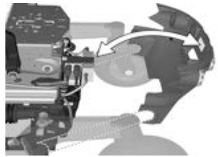
Abbildung 368. Hintere Abdeckung.
