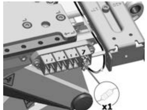
Abbildung 239. Das ICS-Buskabel befindet sich an der siebten Position des Verbinderblocks.
