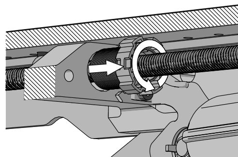
Abbildung 282. Die Kunststoffmutter befindet sich im Schlitten. Der weiß schraffierte Bereich kennzeichnet einen Schnitt durch die Teile, damit Sie eine bessere Sicht haben.
