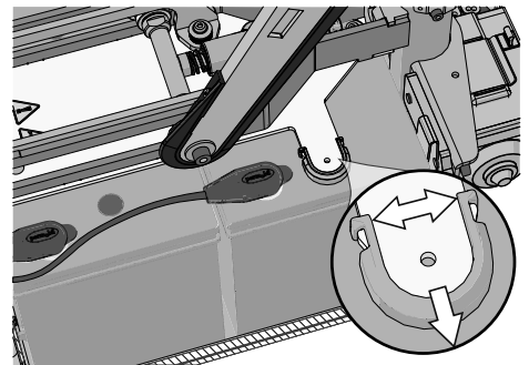
Abbildung 344. AP-Höhenverstellung Batteriepolschutz.
