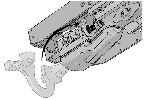
Abbildung 317. Setzen Sie die Halterung wieder ein.
