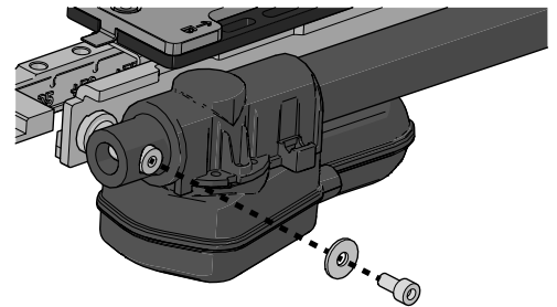
Abbildung 47. Vordere Befestigung der Stellvorrichtung.
