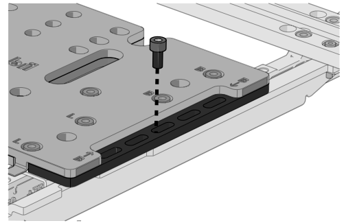
Abbildung 65. Die Schraube, welche die Vorderseite der Stellvorrichtungshalterung sichert.
