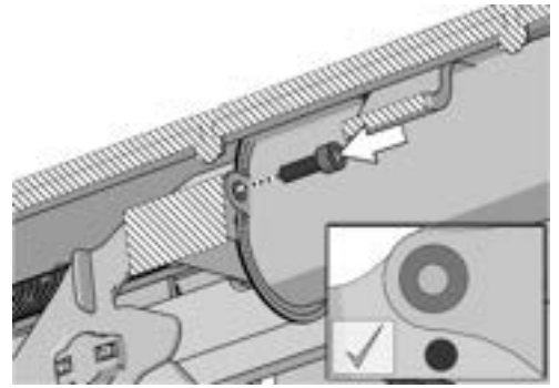
Abbildung 296. Verwenden Sie die obere Öffnung im Schlitten.
