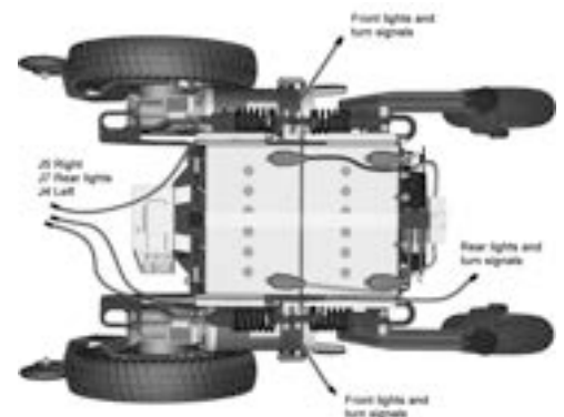
Abbildung 446. Beleuchtungsverkabelung.
