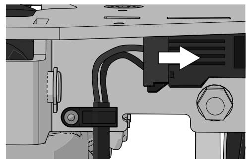
Abbildung 299. Schließen Sie das Kabel der Stellvorrichtung an.
