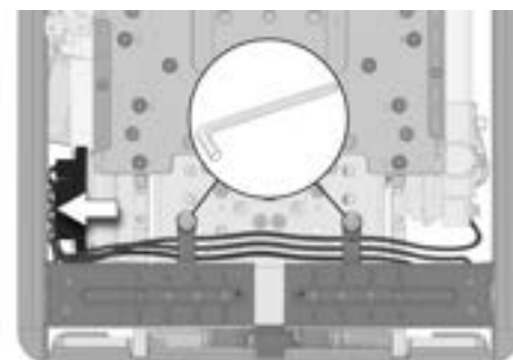
Abbildung 78. Stellvorrichtung Rückenlehne Verkabelung.
