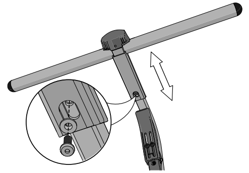
Abbildung 158. Verwenden Sie die M4x10-Schraube, um den vorderen Rahmen zu sichern.
