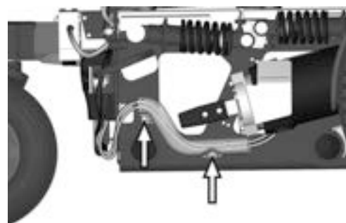
Abbildung 420. Entfernen Sie die Kabelabdeckung.
