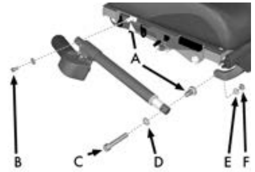
Abbildung 127. Die REAC-Stellvorrichtung für die Beinstütze wird von zwei Verschraubungen (B) und (C) gehalten.
