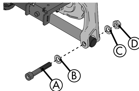
Abbildung 59. Hintere Befestigung der Stellvorrichtung.
