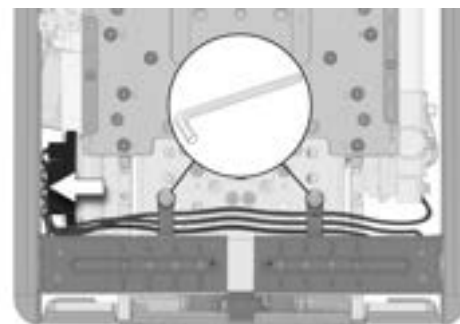
Abbildung 52. Stellvorrichtung Rückenlehne Verkabelung.
