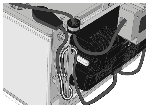
Abbildung 363. Schließen Sie das Kabel vom linken, hinteren Batteriepol am zugehörigen Kabelhalter an, siehe Abbildung.
