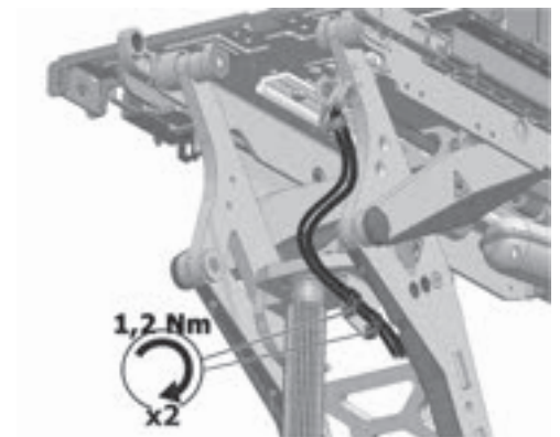
Abbildung 470. Das Buskabel ist in den zwei Kabelhalterungen auf dem unteren Teil des AP-Höhenverstellungsarms angebracht.
