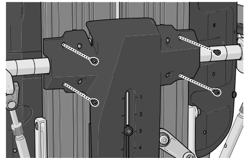
Abbildung 21. Die Anbringungsstellen der vier Schrauben, die die Kunststoffabdeckung sichern.
