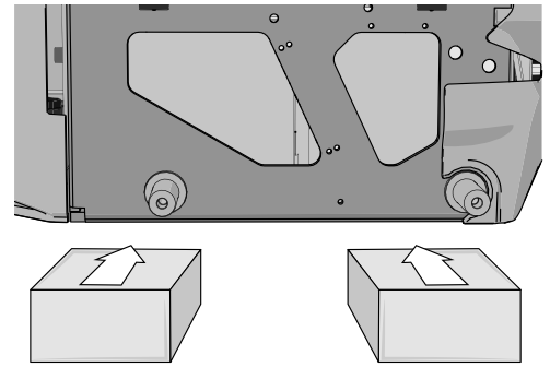
Abbildung 427. Verwenden Sie jeweils zwei Blöcke auf jeder Seite des Fahrgestellkastens. Zur besseren Darstellung wurden die Räder in dieser Abbildung entfernt.
