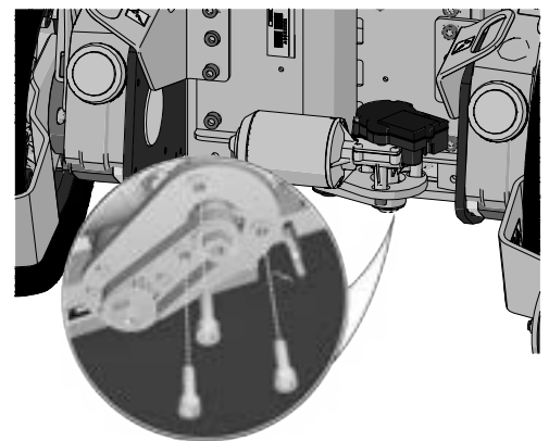
Abbildung 244. Der Motor ist mit drei Schrauben befestigt.
