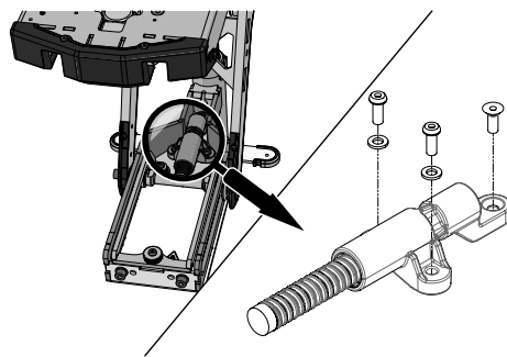
Abbildung 346. Die montierte Federeinheit ist mit drei Schrauben und Unterlegscheiben befestigt.
