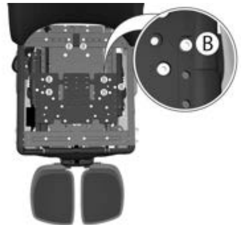
Abbildung 209. Die Position des hinteren Abschnitts des Sitzrahmens (Rückenlehnenposition) wird mit sieben Schrauben gehalten, die hier mit dem Buchstaben B markiert sind.
