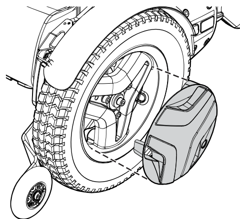
Abbildung 389. Die Radkappe rastet ein, wenn sie sich an ihrem Platz befindet.
