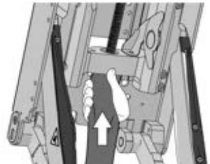
Abbildung 295. Unterseite der oberen Platte.
