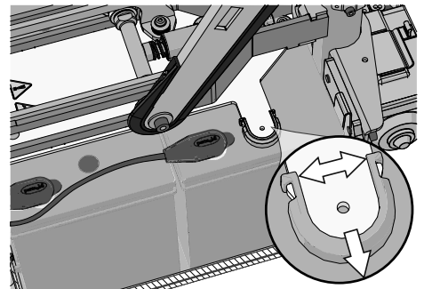
Abbildung 345. AP-Höhenverstellung Batteriepolschutz.
