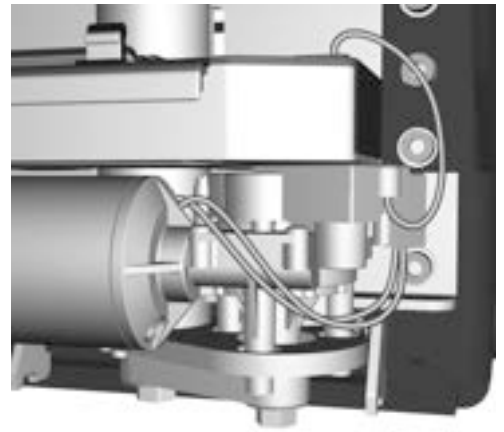
Abbildung 248. Verbinden Sie das Motorkabel mit dem ICS-Mastermodul.
