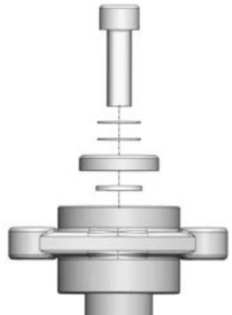
Abbildung 406. Beachten Sie die Montager Reihenfolge der verschiedenen Unterlegscheibentypen.
