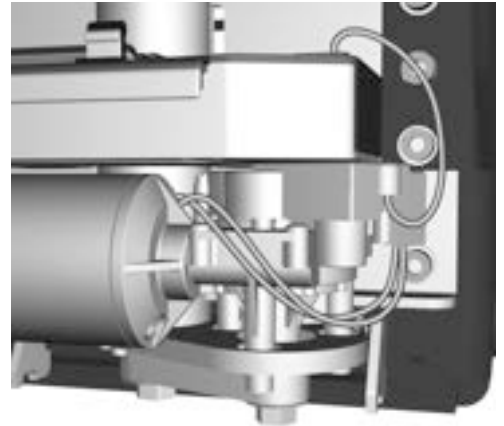
Abbildung 240. Trennen Sie das Höhenverstellungsmotorkabel vom ICS-Mastermodul.
