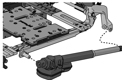
Abbildung 69. Montieren Sie die Rückenlehnen-Stellvorrichtung.
