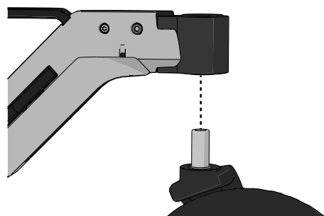
Abbildung 434. Radgabel.
