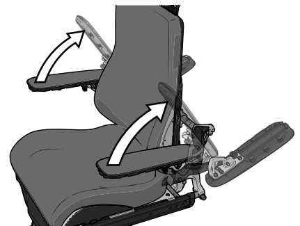
Abbildung 88. Die Armlehnen sind gemeinsam mit dem Armlehnscharnier nur durch die zwei Traversen am Sitz angebracht.
