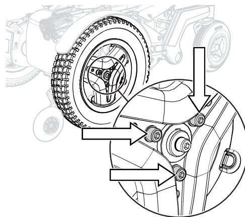
Abbildung 388. Verwenden Sie einen Drehmomentschlüssel, um die Schrauben anzuziehen.
