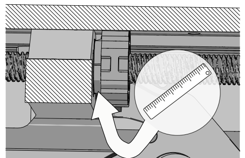
Abbildung 287. Es ist sehr wichtig, dass zwischen Polymermutter und Schlitten eine Lücke vorhanden ist.
