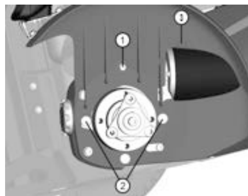
Abbildung 201. Der vordere Kotflügel ist mit einer Schraube (1) und zwei Befestigungspunkten (2) an der Unterseite angebracht.
