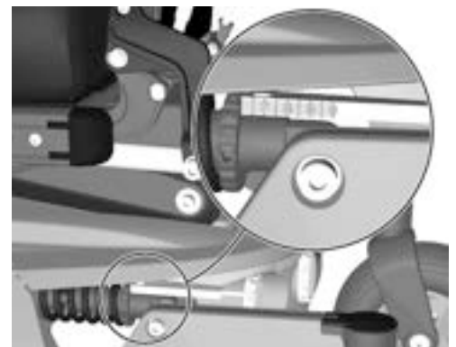
Abbildung 546. Messen Sie die Federkraft-Einstellung der Stoßdämpfer.
