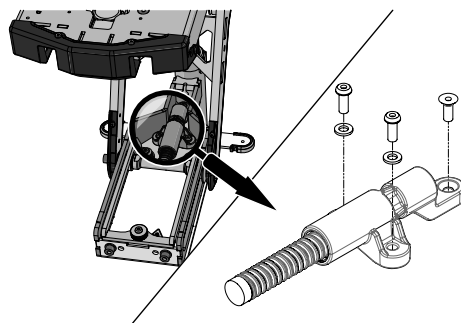
Abbildung 347. Die montierte Federeinheit ist mit drei Schrauben und Unterlegscheiben befestigt.
