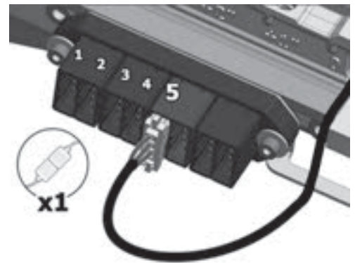
Abbildung 333. Das Kabel für den Sitzneigungsmotor befindet sich an der fünften Position des Verbinderblocks.
