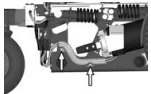
Abbildung 378. Die Kabel von Antriebsmotor und Magnetbremse werden mit einer Kabelabdeckung an ihrem Anbringungsort gehalten.
