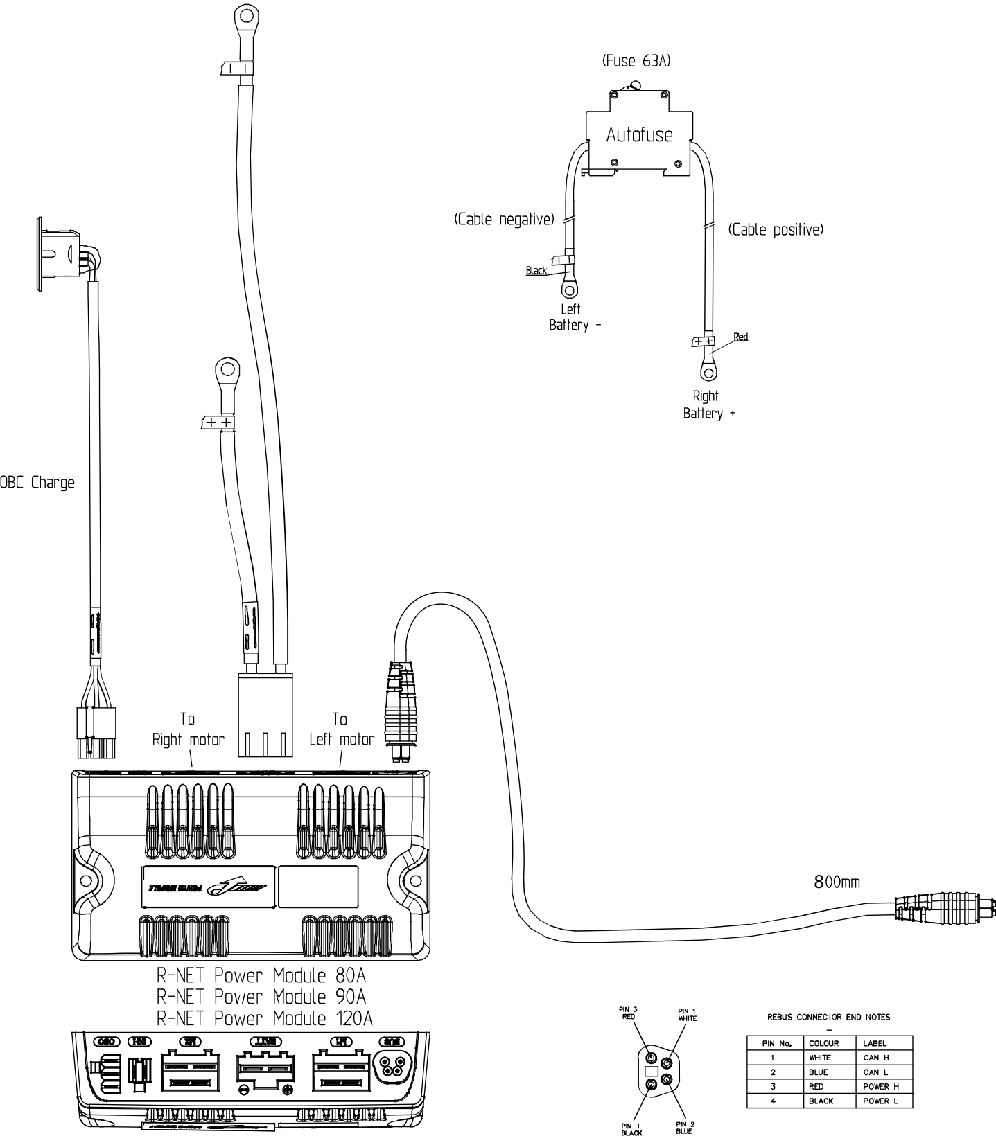
Abbildung 3. Schaltplan Fahrgestellkasten (1 / 2).
