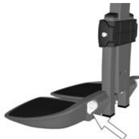
Abbildung 173. Das Metallendstück der Reibungsbremse befindet sich ordnungsgemäß in der vorgesehenen Öffnung in der Fußplatte.
