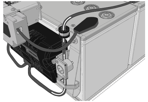
Abbildung 364. Schließen Sie das Kabel vom rechten, vorderen Batteriepol am zugehörigen Kabelhalter an, siehe Abbildung.
