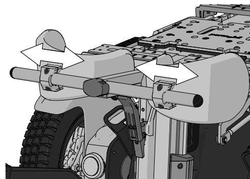
Abbildung 162. Es sollte problemlos möglich sein, die Halterungen zu verschieben, lösen Sie anderenfalls die Schrauben noch mehr.
