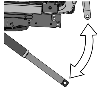
Abbildung 42. Die hintere Befestigung der Stellvorrichtung ist jetzt gelöst.
