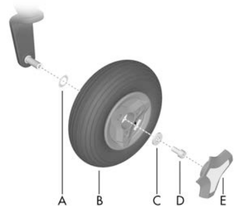
Abbildung 397. Zusammenbauen der Felge.
